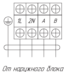
Клеммный терминал внутреннего блока
