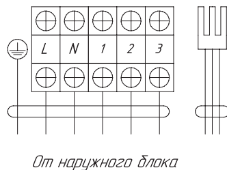
Клеммный терминал внутреннего блока
